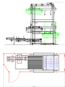
Vista en planta y alzado
