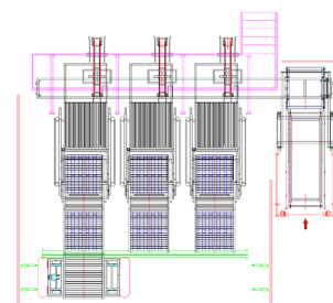
Configuración de sistema totalmente automatizado
